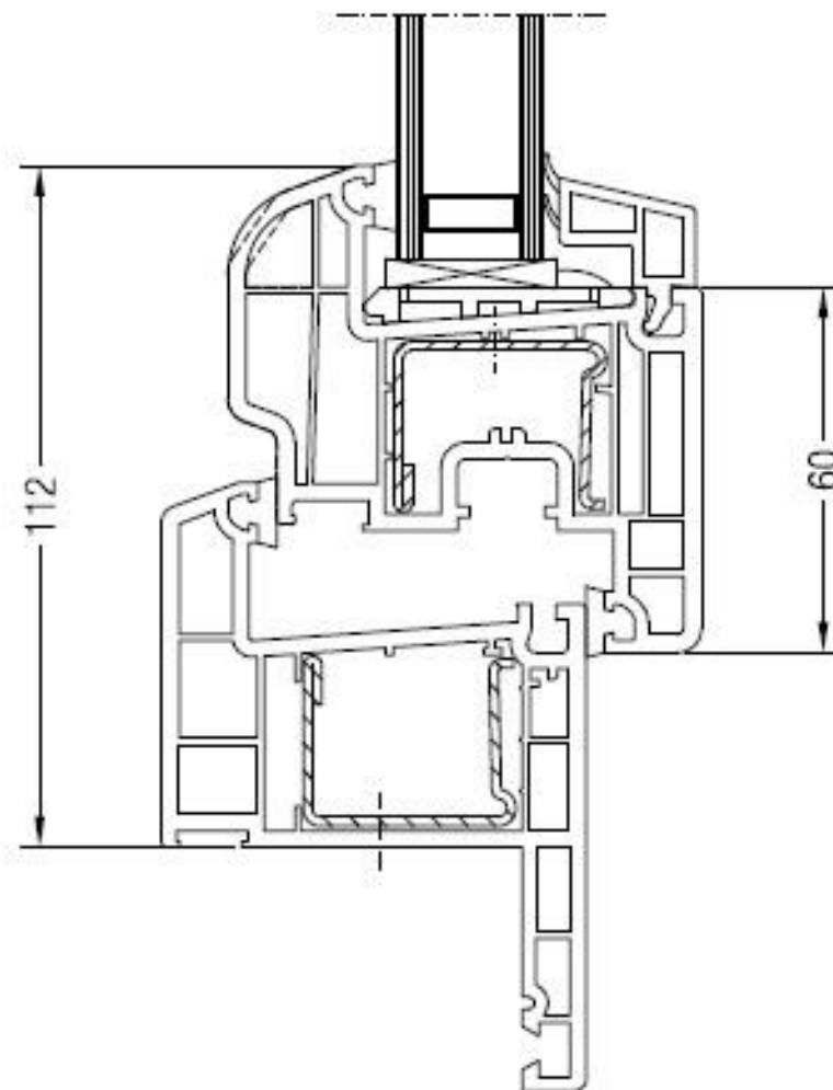
Sezione nodo Brillant 70 telaio Z ( aletta da 40 mm ) – anta arrotondata
