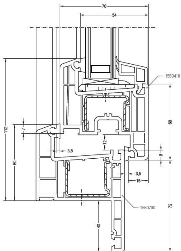
Sezione nodo Brillant 70 telaio Z ( aletta da 40 mm ) – anta dritta
